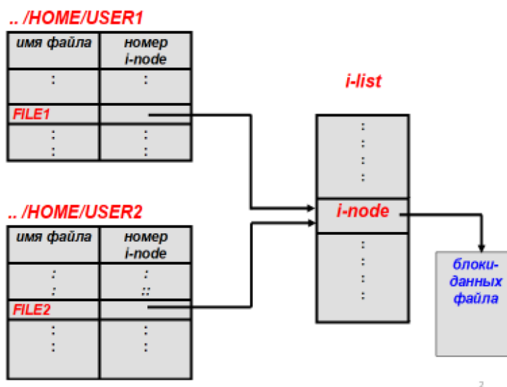
Рисунок 2. Жёсткие ссылки на атрибуты и данные файла
