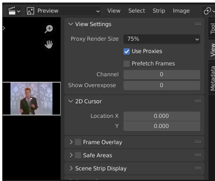
Рис. 13. Окно Properties для установки Proxy size
